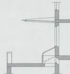
Querschnitt Terrasse
